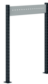
MONTANTS DE SUPERSTRUCTURE hauteur 1200 avec traverses pour établi L. 750 / 1000 / 1200 / 1500 / 1800 / 2000 mm (2 ou 3 montants)
